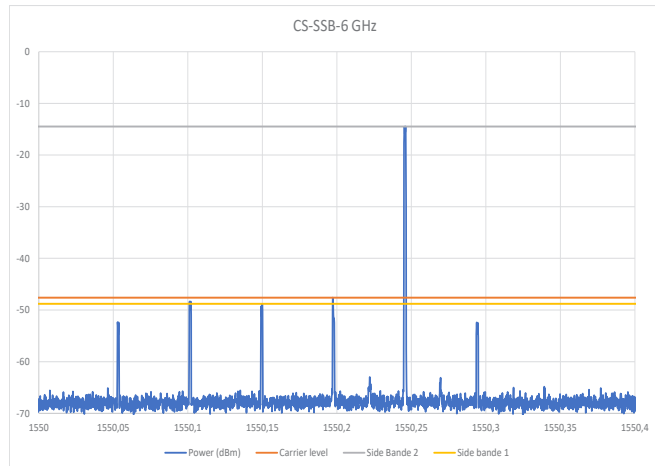
1550 nm - 6 GHz - CS-SSB
