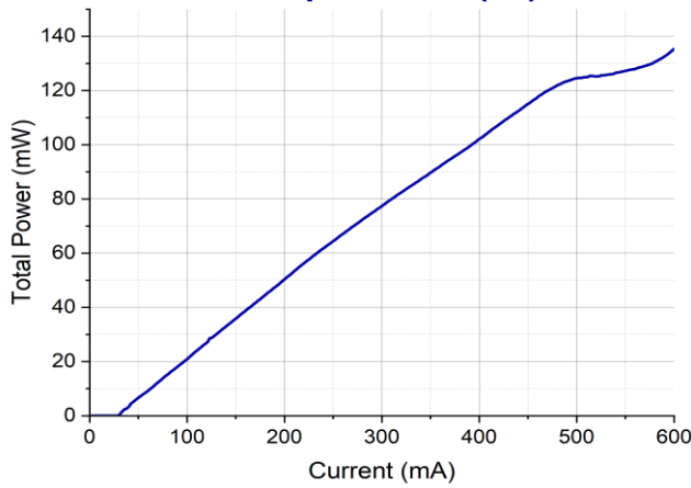
Total Output Power (L-I)
