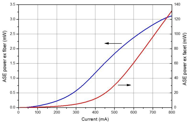
ASE power
