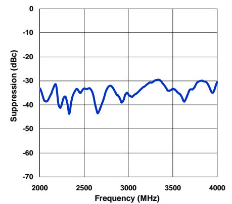
Sideband Suppression
