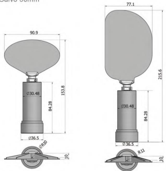
UltraGalvo 50mm
