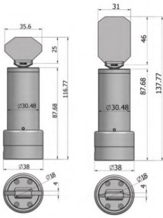
ExtraGalvo 20mm
